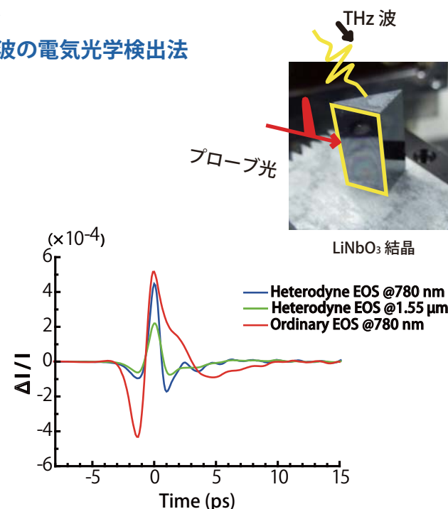
Si プリズム結合 LiNbO 3 結晶 (上図) を用いた THz 波のチェレンコフ位相整合 & ヘテロダイン EO サンプリング検出波形
