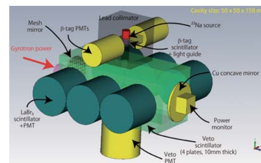
計測装置図
