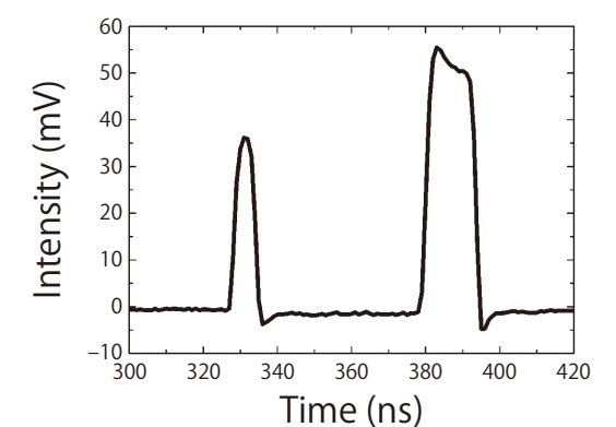
光駆動半導体スイッチングデバイスによりコヒーレンシーを保ったまま 10 ns、20 ns に超短パルス化された 154 GHz ジャイロトロン出力
