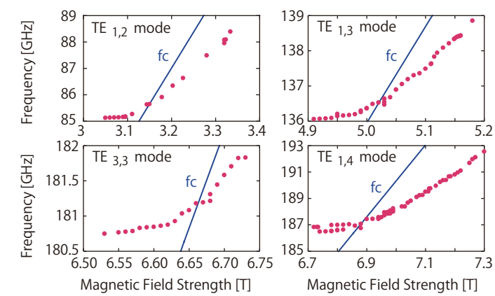
Gyrotron FU CW XA の発振周波数の変化
